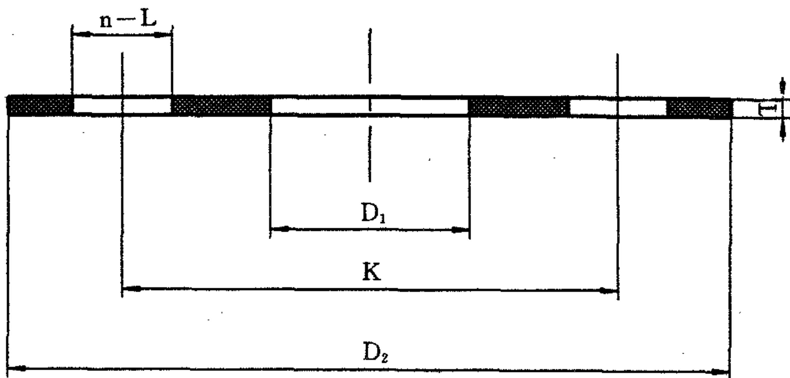
a. FF型(全平面)
