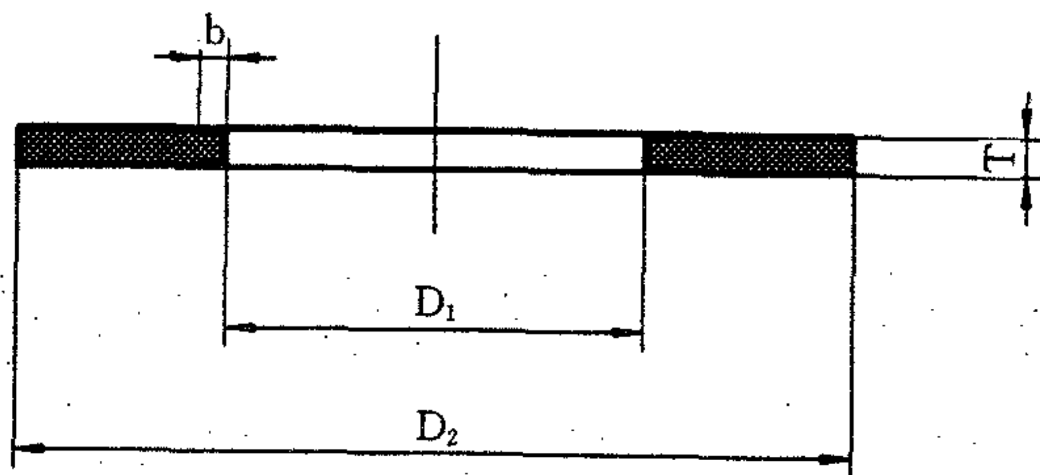
c. RF-E型(突面, 带内包边)
