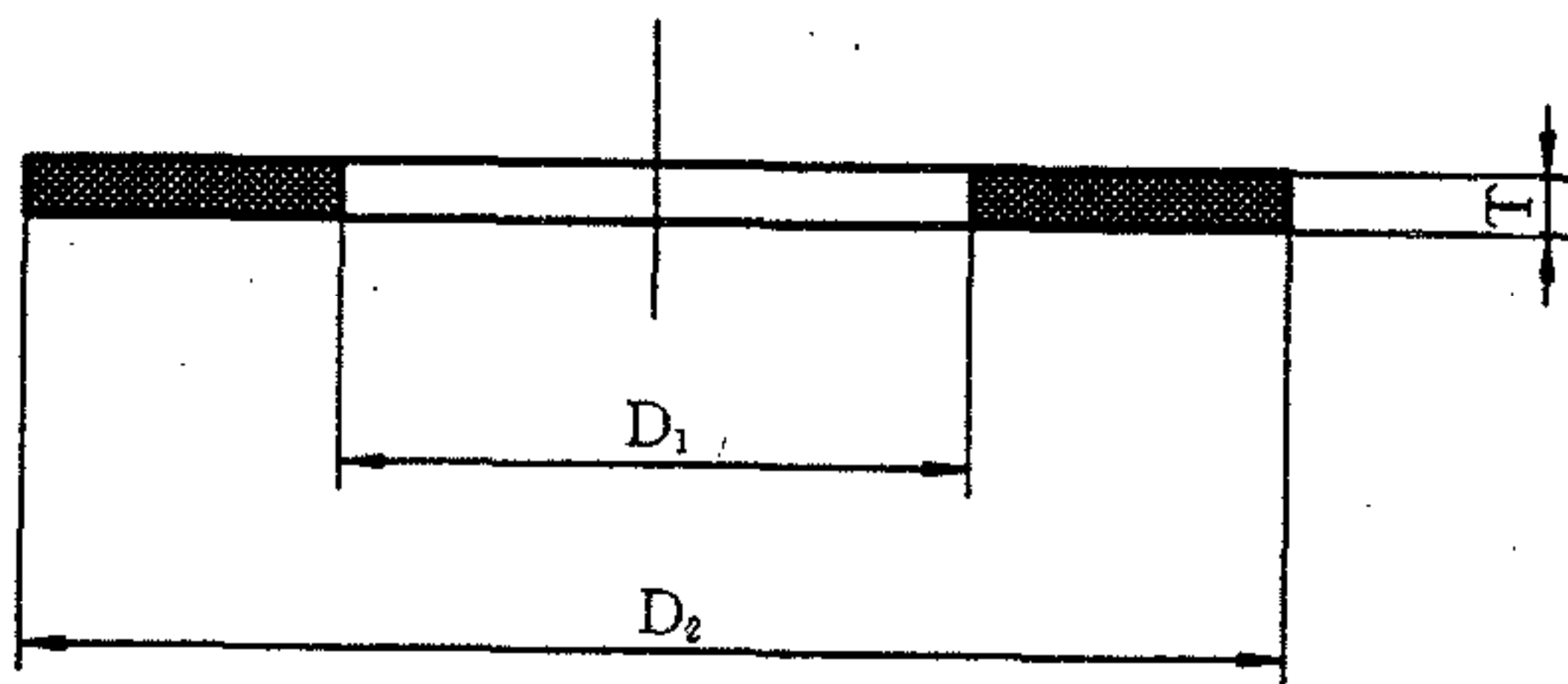
b. RF、MFM、TG型(突面、凹凸面、榫槽面)
